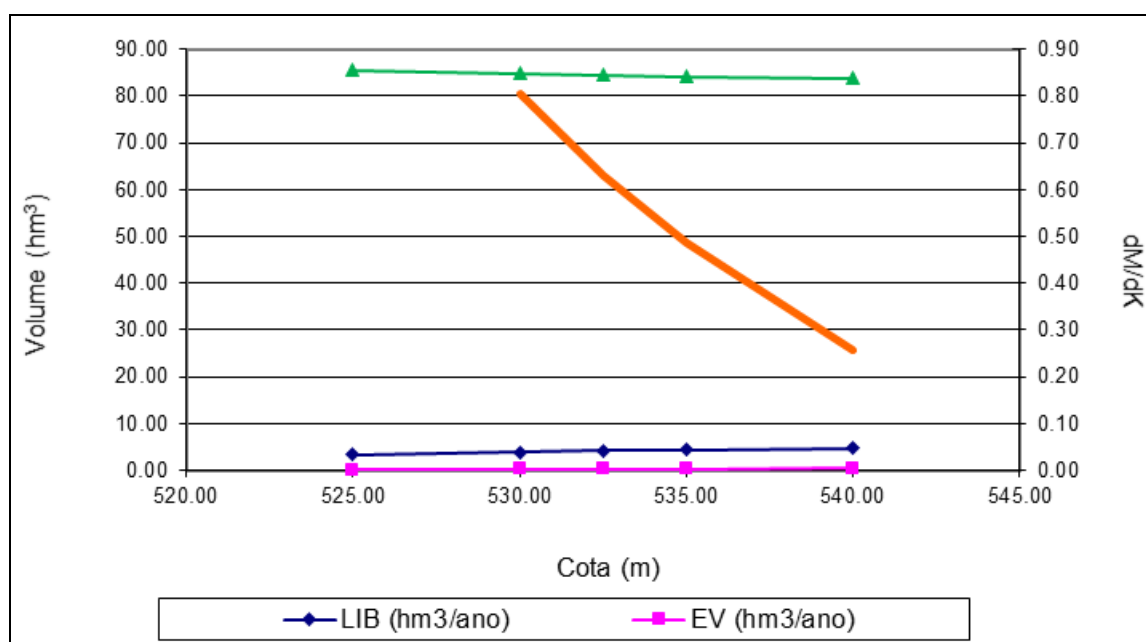
Figura 2.24 – Curvas de regulação da barragem Beré (Resolução direta da equação do balanço hídrico – Garantia de 99%)
