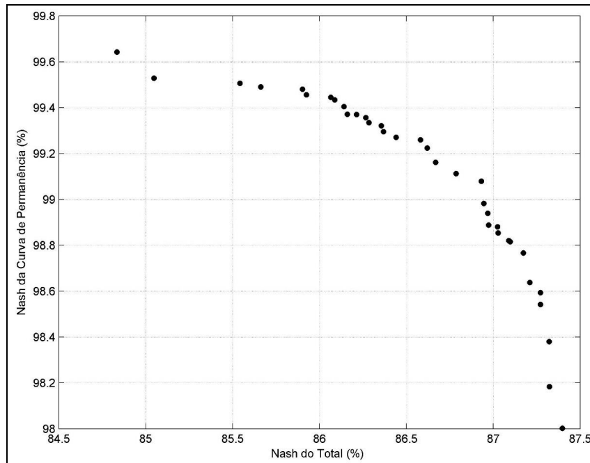
Figura 2.22 – Calibração do modelo MODHAC para o posto 36250000
