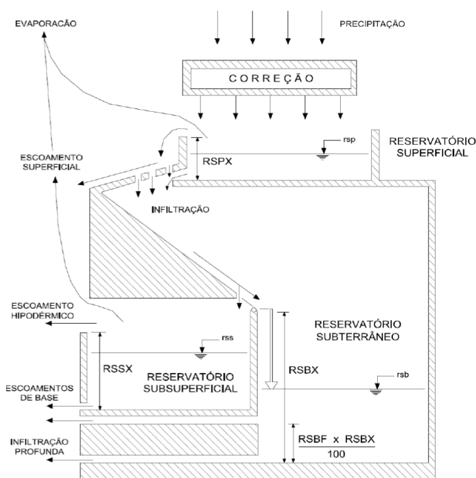
Figura 2.21 – Representação do modelo MODHAC (Lanna, 1997)
