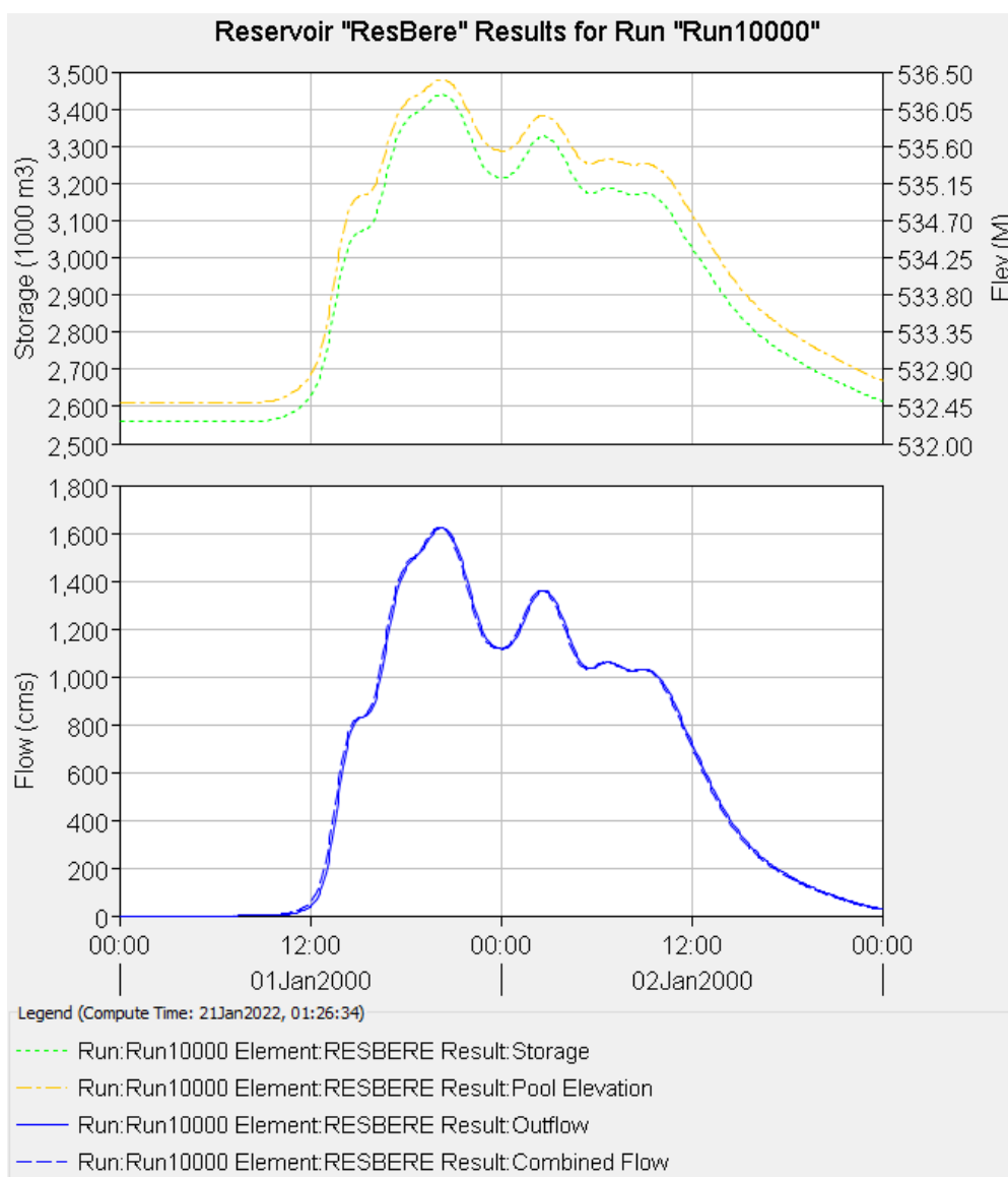
Figura 2.28 – Hidrograma total afluente à barragem Beré (Tr = 10.000 anos)
