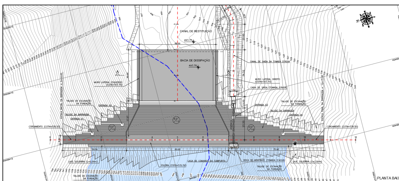
Figura 3.8 – Layout geral da barragem
