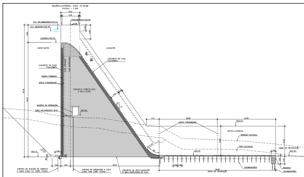
Figura 3.10 – Seção tipo da barragem (submersível), vertedouro e bacia de dissipação
