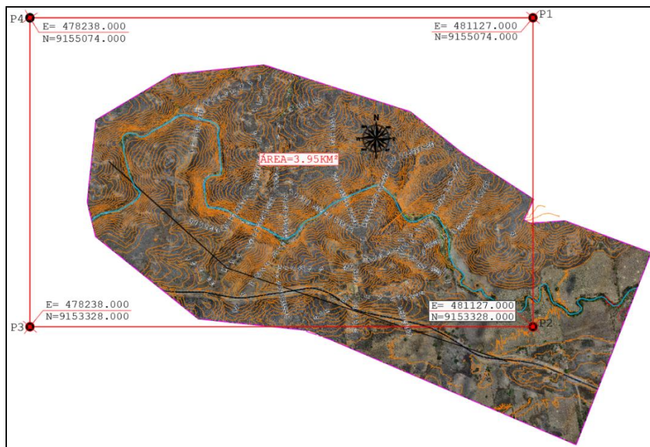
Figura 2.9 – Levantamento Aerofotogramétrico da Segunda Área Voada
