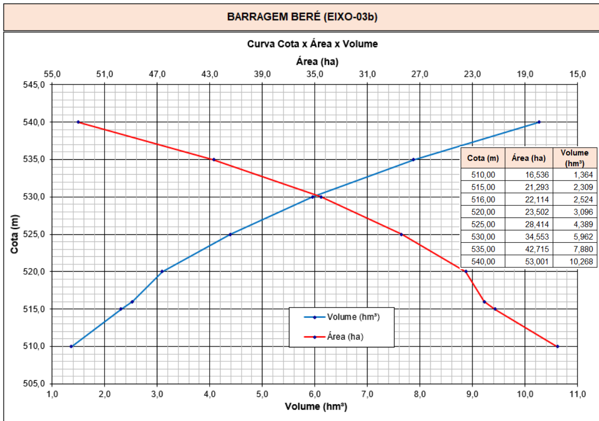
Figura 3.7 – Curvas cota x área x volume do Eixo 03b
