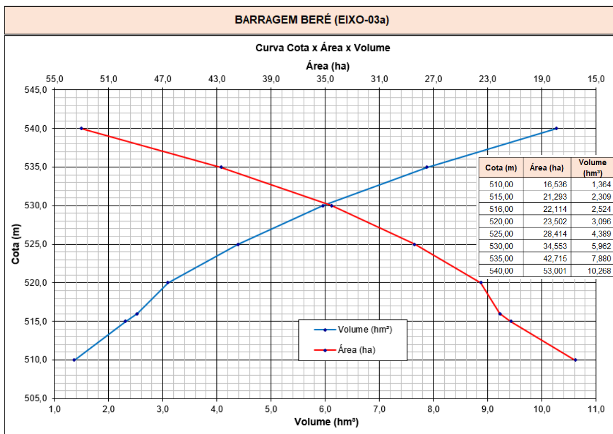
Figura 3.6 – Curvas cota x área x volume do Eixo 03a
