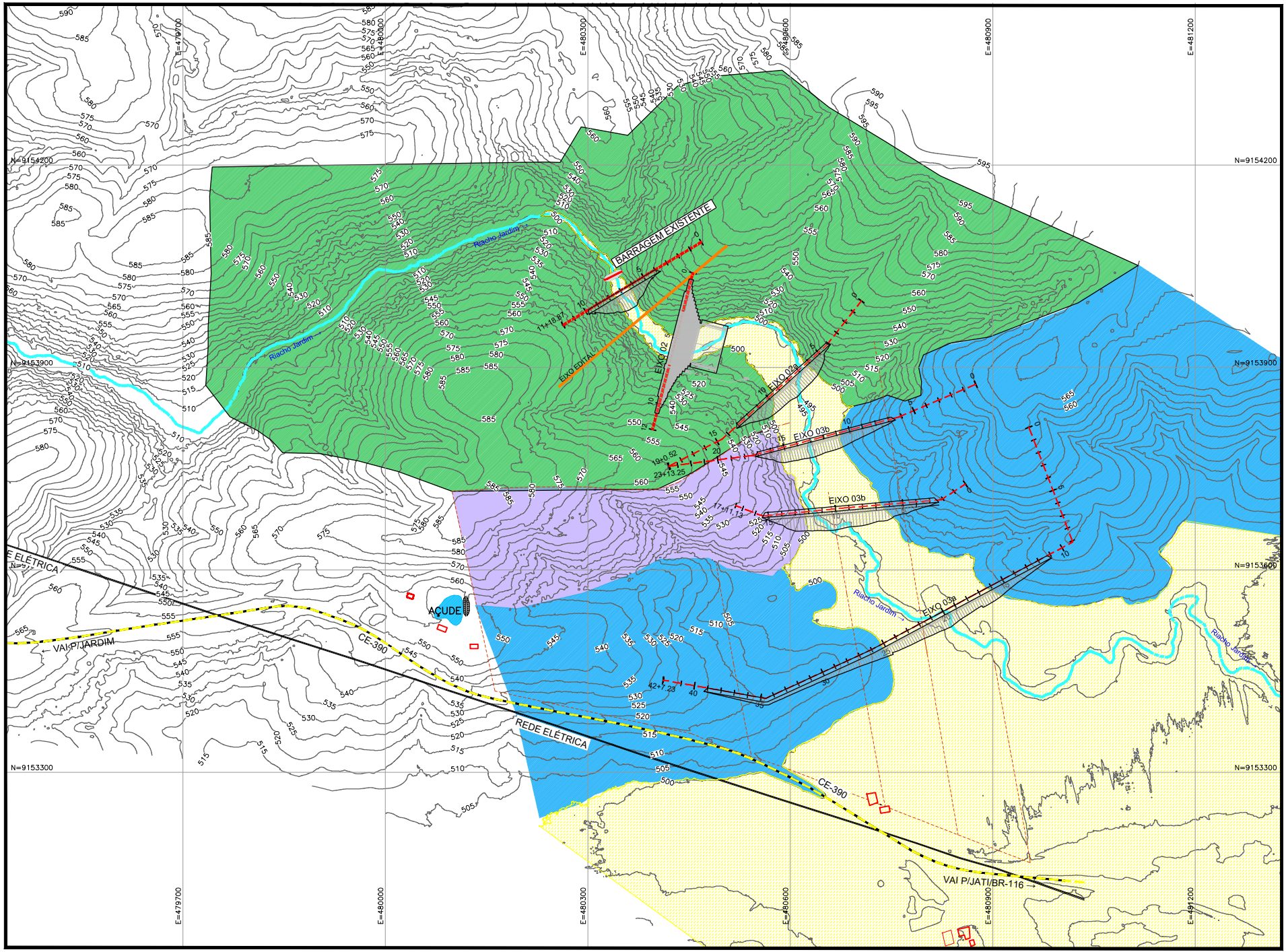
Figura 2.13 – Geologia Local da Barragem Beré
