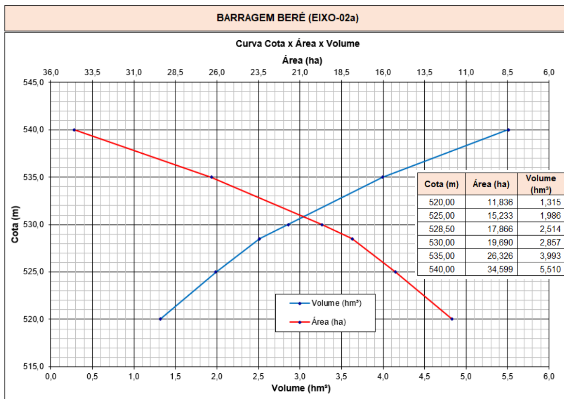
Figura 3.4 – Curvas cota x área x volume do Eixo 02a
