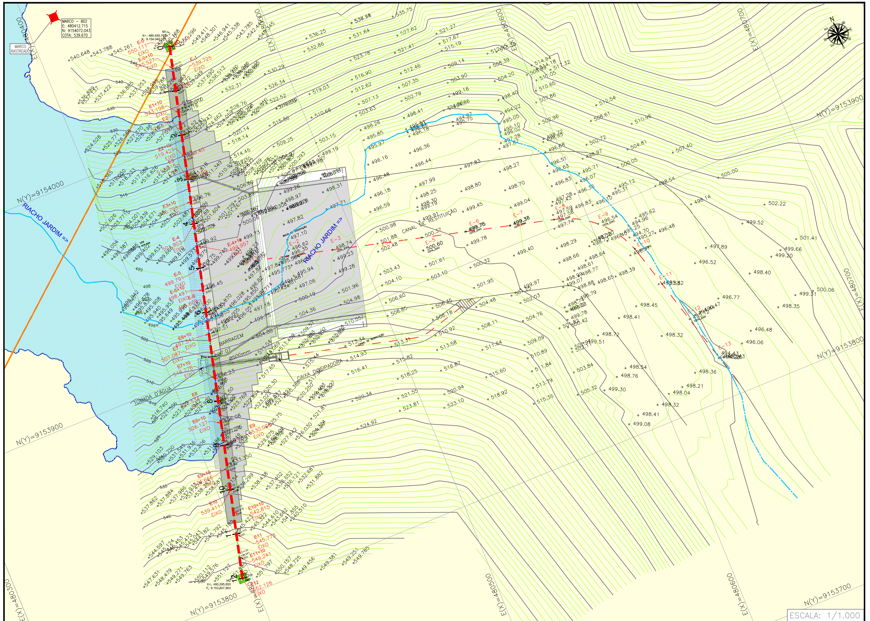
Figura 2.10 – Levantamento Topográfico do Sítio da Barragem Beré
