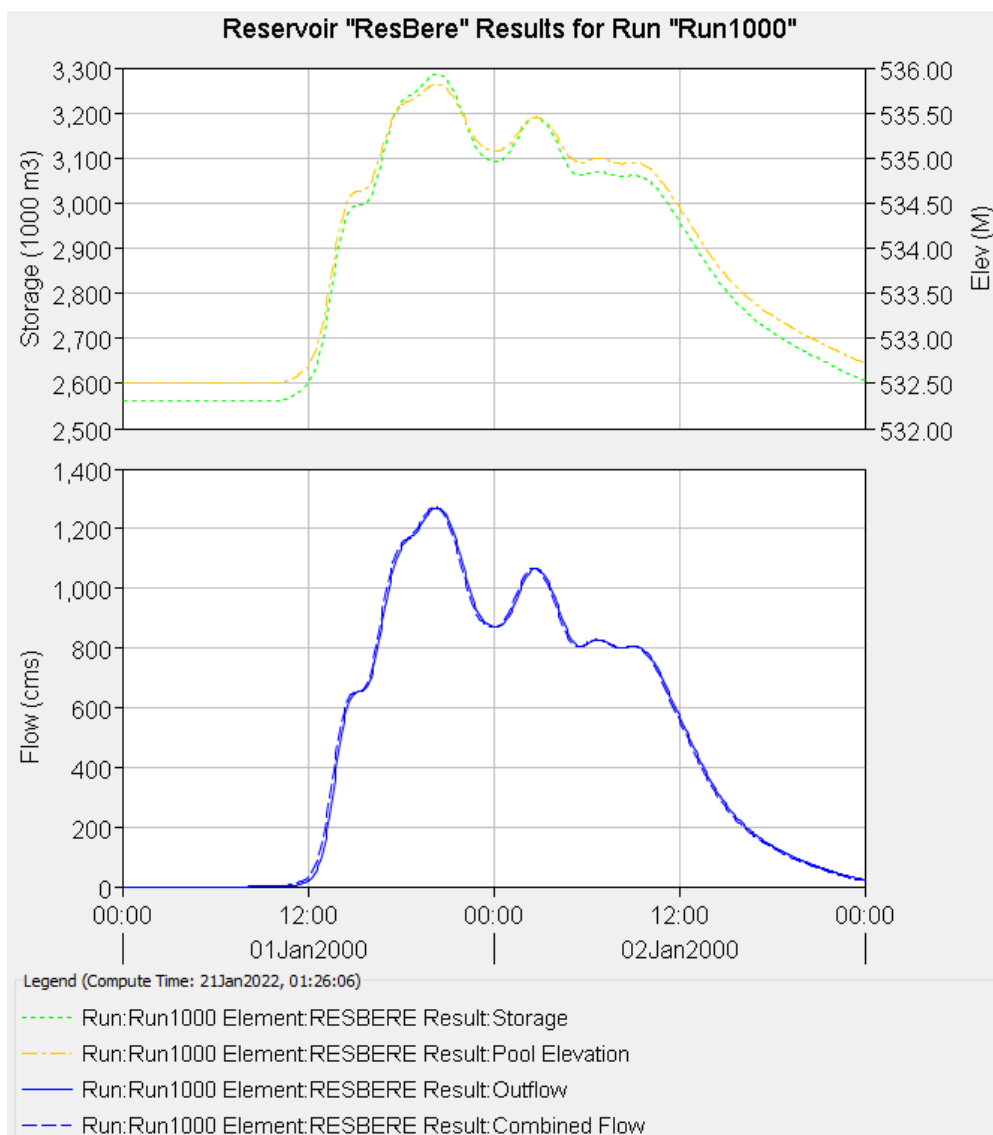
Figura 2.27 – Hidrograma total afluyente à barragem Beré (Tr = 1.000 anos)
