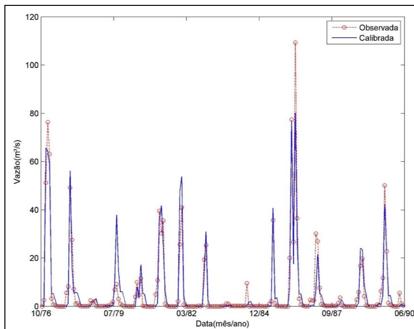
Figura 2.23 – Vazões do modelo MODHAC para o posto 36250000
