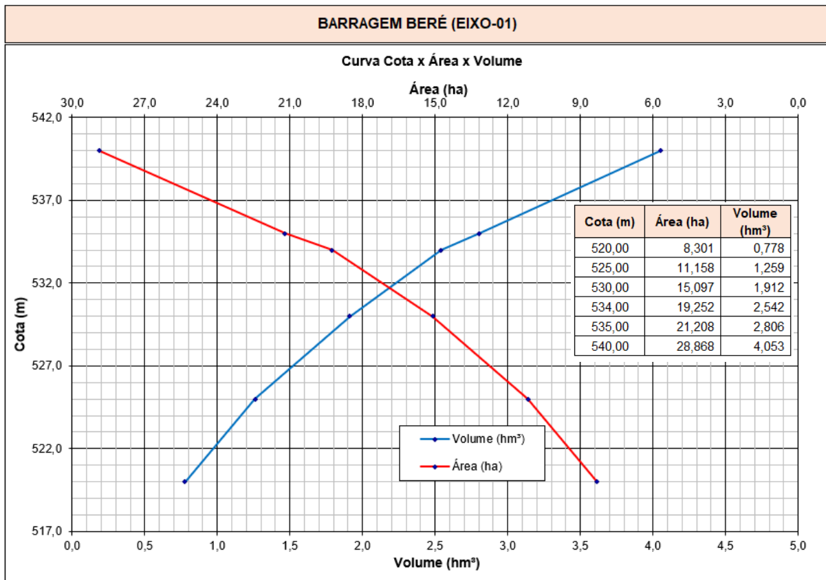
Figura 3.2 – Curvas cota x área x volume do Eixo 01
