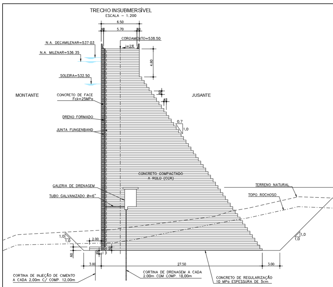
Figura 3.9 – Seção tipo da barragem (insumersível)
