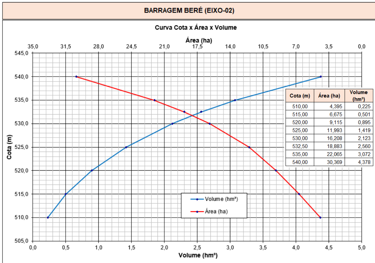
Figura 3.3 – Curvas cota x área x volume do Eixo 02
