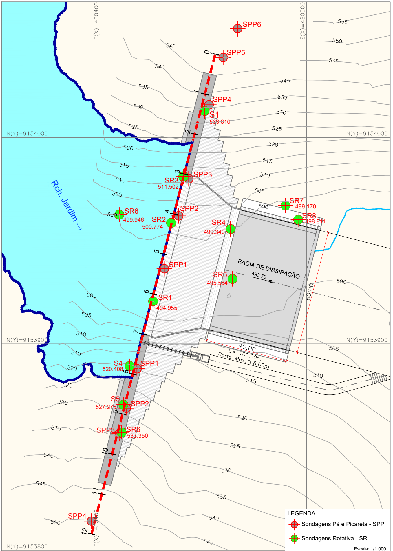
Figura 2.14 – Localização das Sondagens Executadas no Eixo 02 (selecionado)
