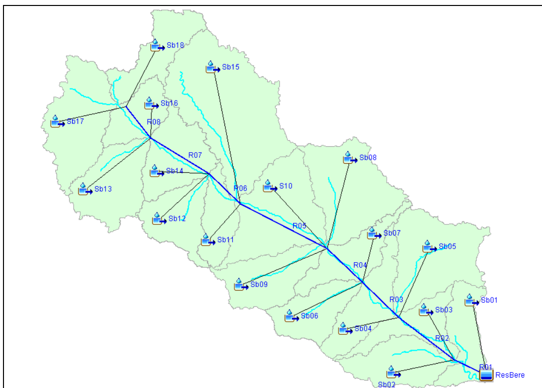
Figura 2.26 – Rede simulada no HEC-HMS
