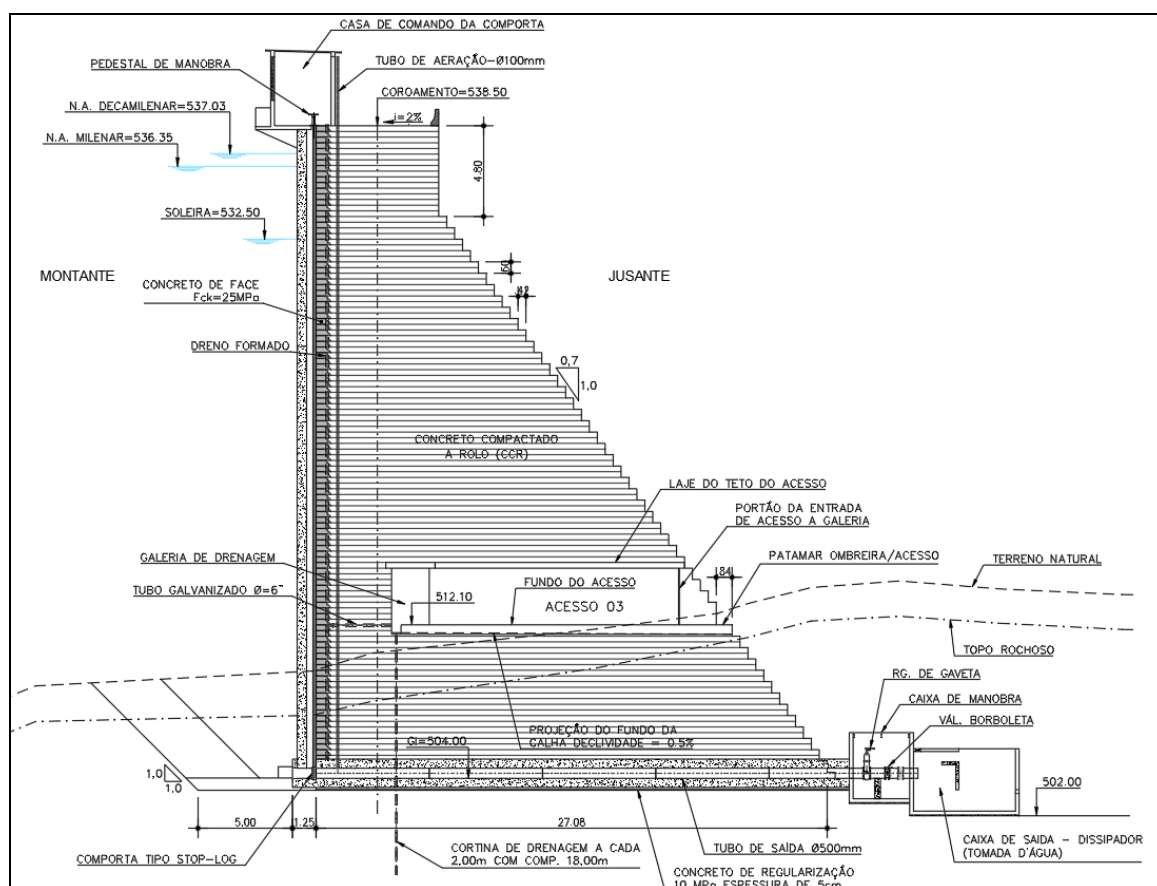
Figura 3.11 – Seção tipo da barragem (insubmersível) tomada d'água
