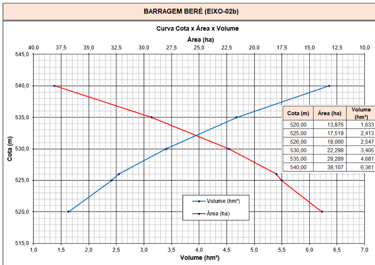
Figura 3.5 – Curvas cota x área x volume do Eixo 02b
